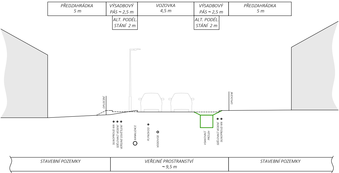
ULIČNÍ PROFIL 2 - UL. MYSLIVECKÁ - MÍSTNÍ OBSLUŽNÁ KOMUNIKACE DVOUPRUHOVÁ OBOUSMĚRNÁ
