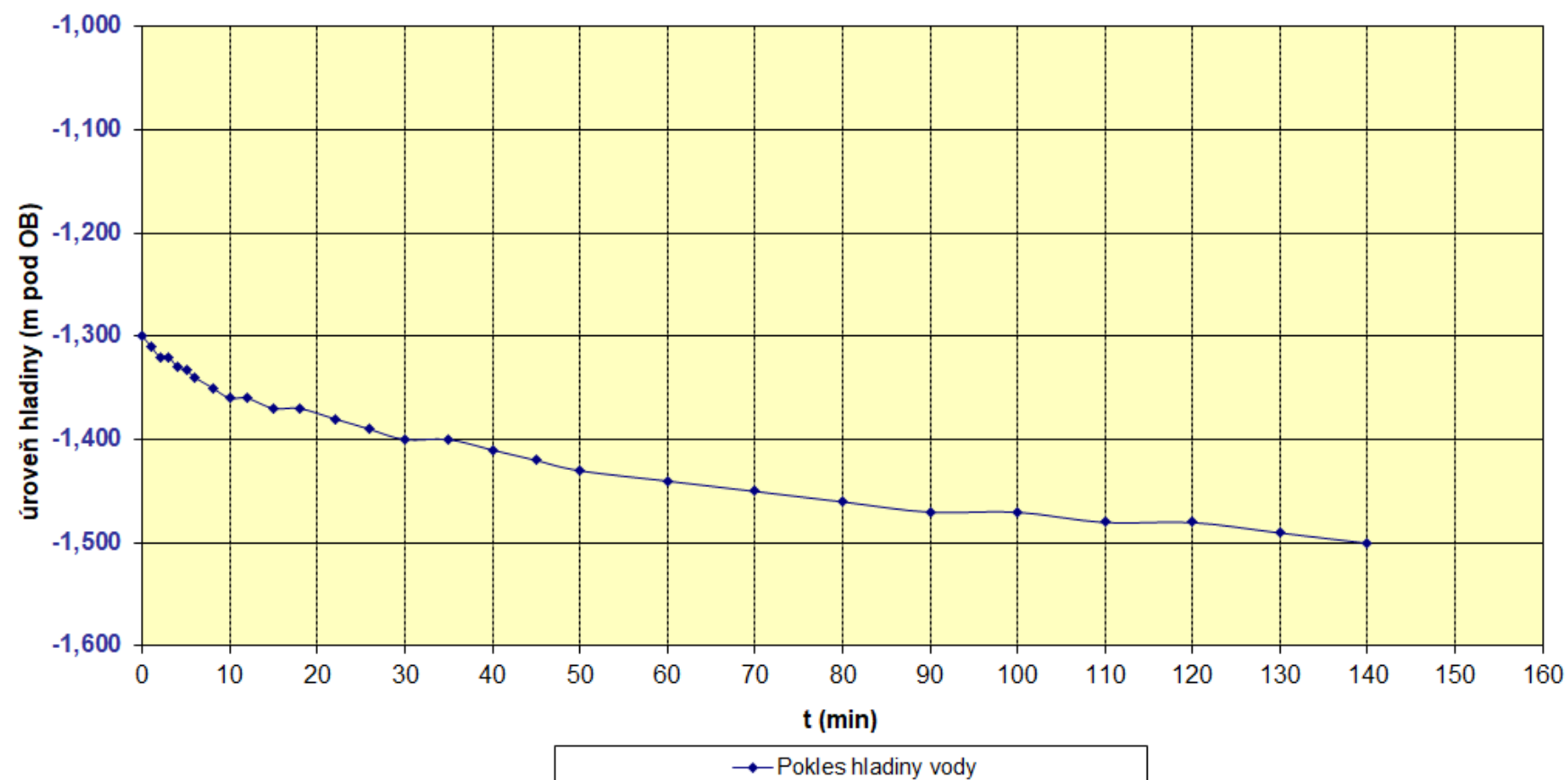
GRAF zasakovací zkoušky v kopané sondě KS-5
