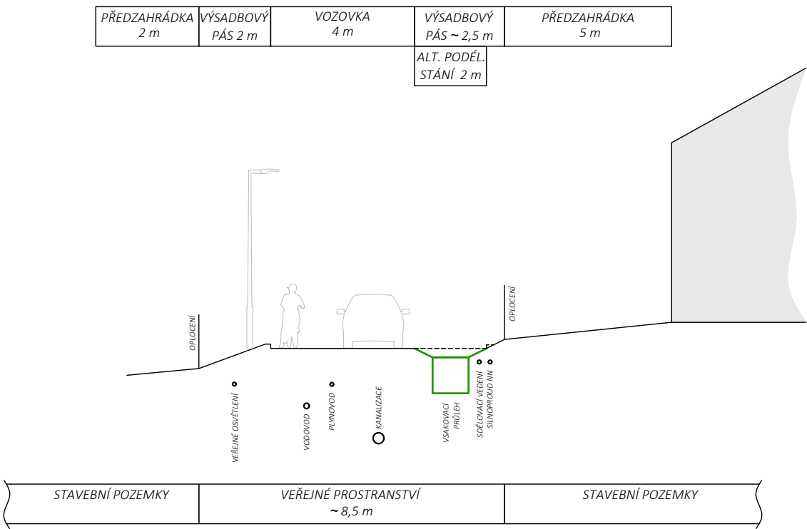
ULIČNÍ PROFIL 3 - MÍSTNÍ OBSLUŽNÁ KOMUNIKACE JEDNOPRUHOVÁ OBOUSMĚRNÁ
