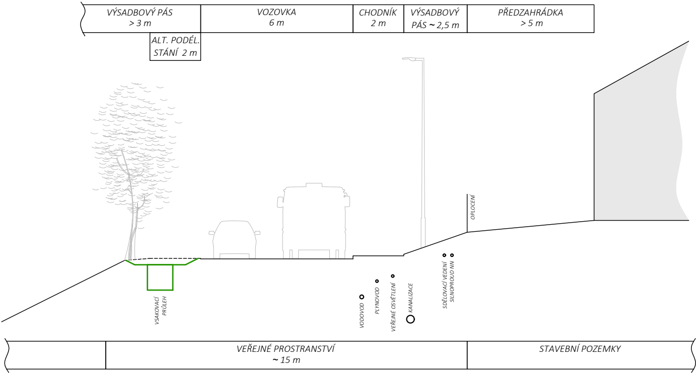
ULIČNÍ PROFIL 1 - UL. DVORSKÉHO - SILNICE DVOUPRUHOVÁ OBOUSMĚRNÁ
