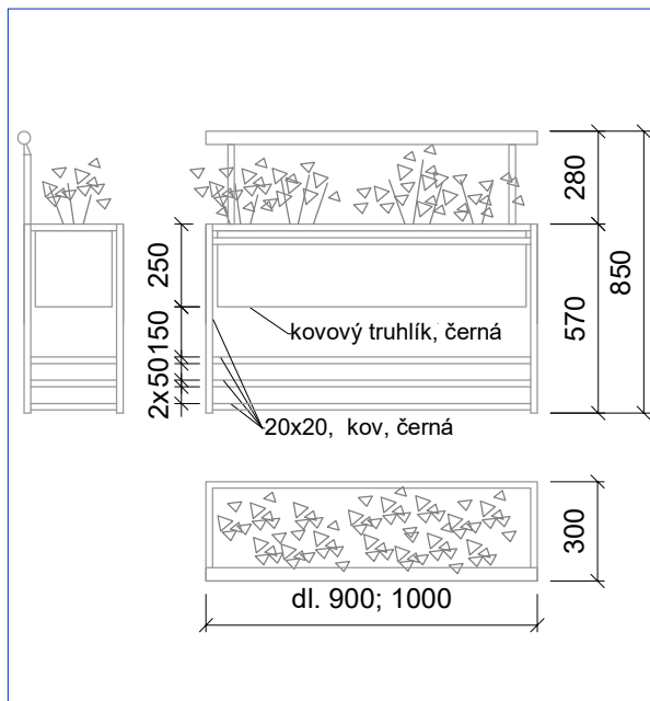
detail - ohrazení - m 1:25
